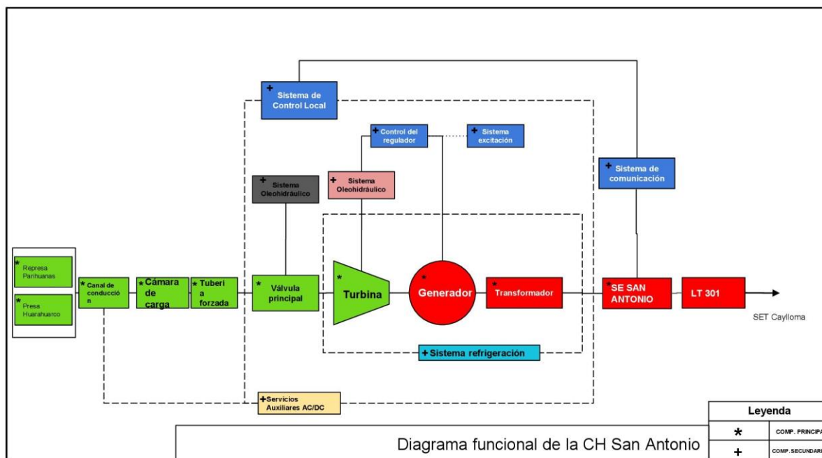
Figura N° 1. Diagrama de flujo de la CH San Antonio
